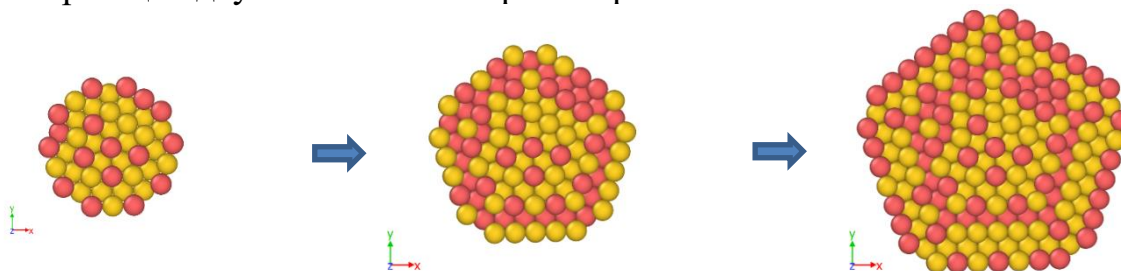
Рис. 1. Послойный рост наночастицы Au-Ag, в разрезе плоскостью (001).
