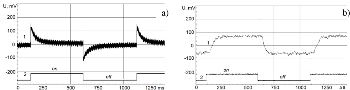
Рис. 3. Характерный пироэлектрический отклик гетероструктуры AlGaN/SiC/Si, полученный на частотах 1 Hz (a) и 1 kHz (b). Стробы (2) иллюстрируют модулированный тепловой поток.
