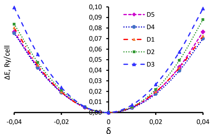
Рис. 1. Кривые разностей полных энергий, \Delta E , в зависимости от приложенных деформаций \delta , возникающих при воздействии матриц искажений D_1 - D_5 [2] на кристаллическую решетку \text{Fe}_7\text{Mo}_6 .
