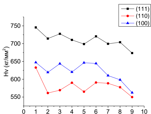
Рис.1. Значения микротвердости монокристалла Ge для кристаллографических плоскостей (111), (100), (110).
