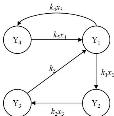
Рис. 1. Граф Темкина механизма паровой конверсии метана на никелевом катализаторе
