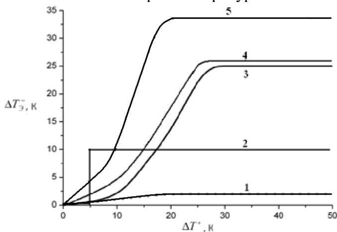
Рис. 1. Графики зависимости перегрева \Delta T^+ от переохлаждения \Delta T_3^- : 1 – для индия; 2 – для олова; 3- для эвтектики Ga-In; 4 – для эвтектики Ga-Sn; 5 – для галлия
