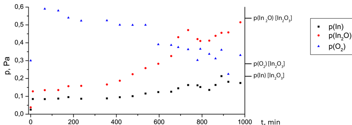
Рис. 1. Парциальные давления компонентов пара над \text{In}_2\text{O}_3 в присутствии Pt. p(\text{In})[\text{In}_2\text{O}_3] , p(\text{In}_2\text{O})[\text{In}_2\text{O}_3] , p(\text{O}_2)[\text{In}_2\text{O}_3] – значения парциальных давлений компонентов пара чистого \text{In}_2\text{O}_3 .
