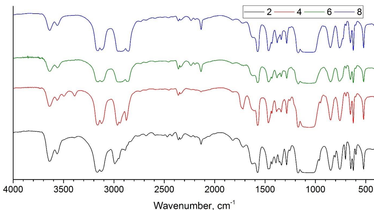
Рис. 1. ИК-спектры ИЖ \text{C}_n\text{MImBF}_4
