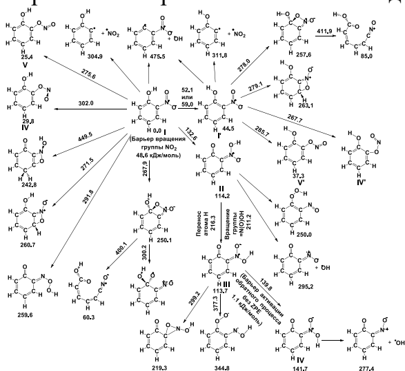
Рис. 1 – Схема термического распада 2-нитрофенола, полученная методом V3LYP/6-31+G(2df,p)*. Рис. 2 – Схема термодеструкции 2-нитрофенола, полученная методом QM_N3*.
