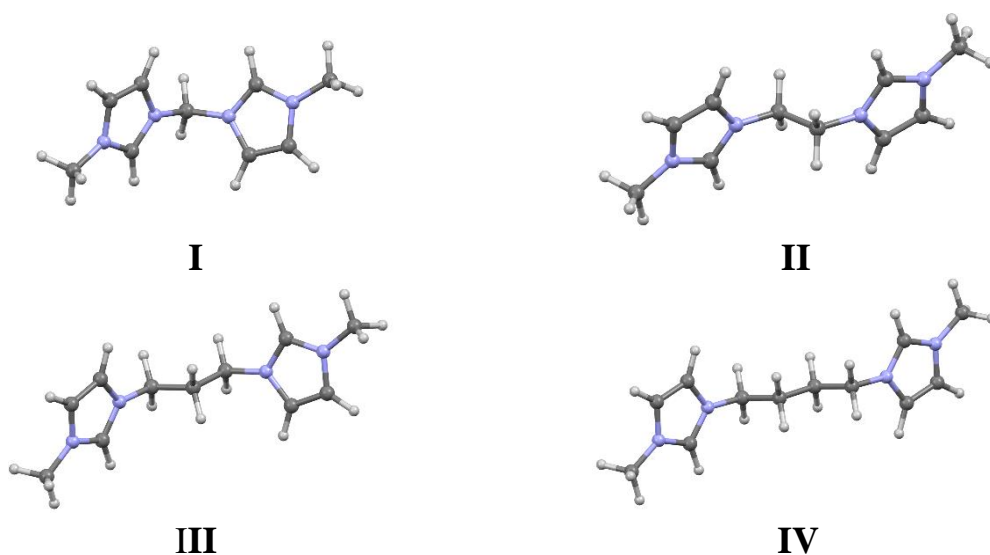
Рис.1. Структуры низколежащих конформеров дикатионов бис(3'-метиylimидазолий-1'-ил)метана ( I ), 1,2-бис(3'-метиylimидазолий-1'-ил)этана ( II ), 1,3-бис(3'-метиylimидазолий-1'-ил)пропана ( III ), 1,4-бис(3'-метиylimидазолий-1'-ил)бутана ( IV ).
