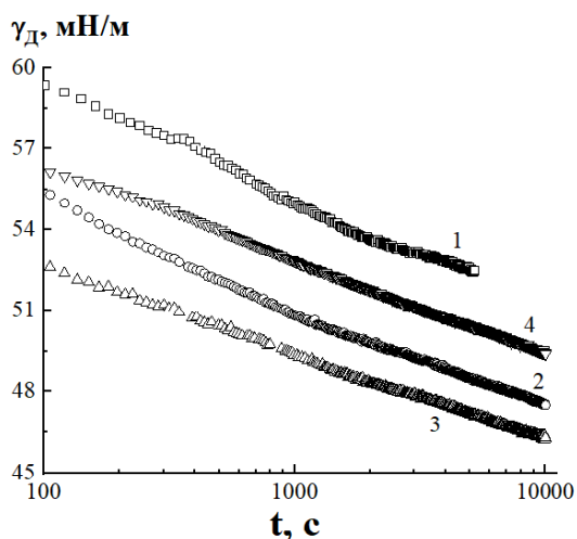
Рис. 1. Изменение динамического поверхностного натяжения растворов солей ГК от времени. 1 – ГН; 2 – ГНГК+пэг-ГНГК+пэг-6000; 3 – ГНГК+гидроперит; 4 – ГНГК+пэг-6000+гидроперит. СПАВ = 0,8%.
