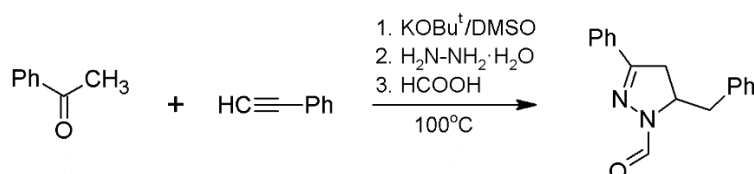
Схема 1. Образование 1-формил-2-пиразолина из ацетофенона, фенилацетилен, гидразина и муравьиной кислоты в системе КОБу t /ДМСО
