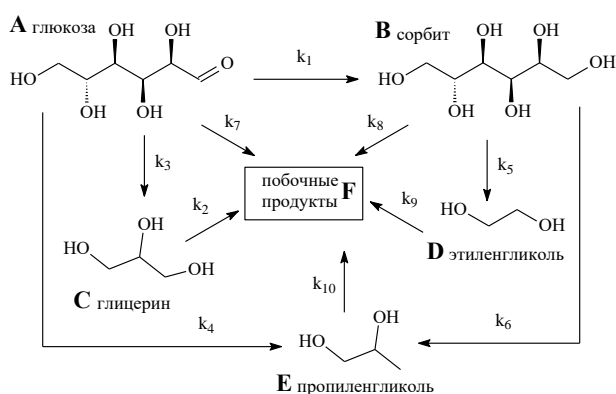
Рис. 1. Схема гидрогенолиза глюкозы до гликолей.
