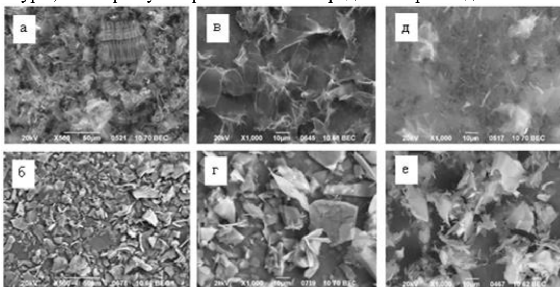
Рис. 1. СЭМ-изображения лиофилизатов суспензий «свежеприготовленных» GO-H (а) и GO-B (б); после повторного приготовления водных суспензий из сухих GO-H (в) и GO-B (г) с механическим перемешиванием; после повторного приготовления водных суспензий из сухих GO-H (д) и GO-B (е) при воздействии ультразвука.
