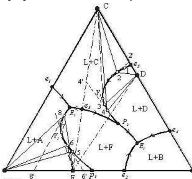
Рис. 1. Точки инверсии Y_1 и Y_2 со сменой типа трехфазной реакции на моновариантных кривых ликвидуса e_5P_2 и p_1E_1 [4, с. 208, рис. 3.64]
