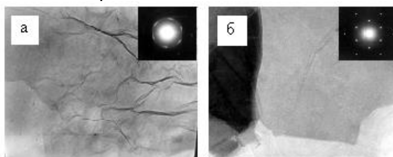
Рис. 2. ПЭМ-микрофотографии частиц GO-H (а) и GO-B (б) (на вкладках соответствующие им электронограммы).
