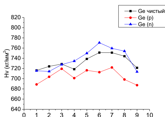
Рис. 2. Значения микротвердости монокристаллов Ge разных типов проводимости.
