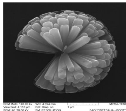
Рис. 3. Массив полусфероподобных ограниченных наностержней
