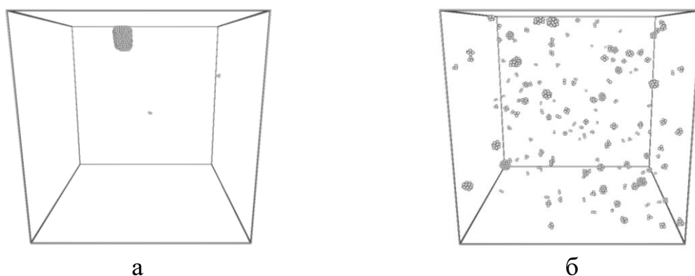
Рис. 2. Примеры конечных конфигураций после 10 млн. шагов моделирования при использовании потенциала сильной связи (а) и метода погруженного атома (б).
