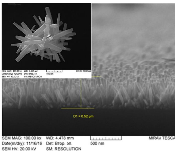
Рис. 1. РЭМ-изображение наностержней ZnO, синтезированных без добавления дополнительных прекурсоров.
