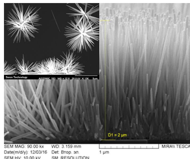
Рис. 2. РЭМ-изображение наностержней ZnO, синтезированных с добавлением аммиачной воды и полиэтиленимина в ростовой раствор.
