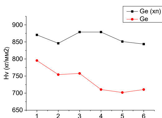
Рис. 3. Изменение значений микротвердости монокристаллов Ge после химической полировки.
