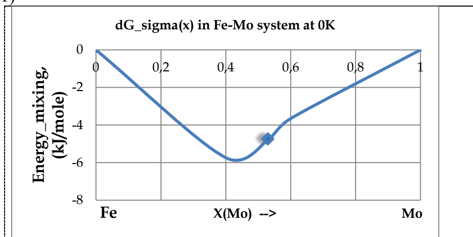
Рис. 1. Зависимость энергии смешения \sigma – фазы относительно \sigma - фаз чистых компонентов в зависимости от состава x(Mo) \sigma - фазы системы Fe-Mo.
