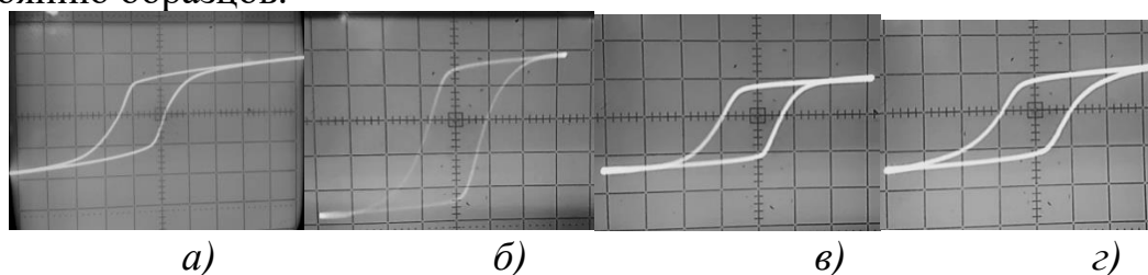
Рис.1. Осциллограммы петель диэлектрического гистерезиса, полученные для образцов BaTiO 3 : Nb 5+ : а – С = 0; б – С = 0,1; в – С = 0,3; г – С = 0,9 мол. %.
