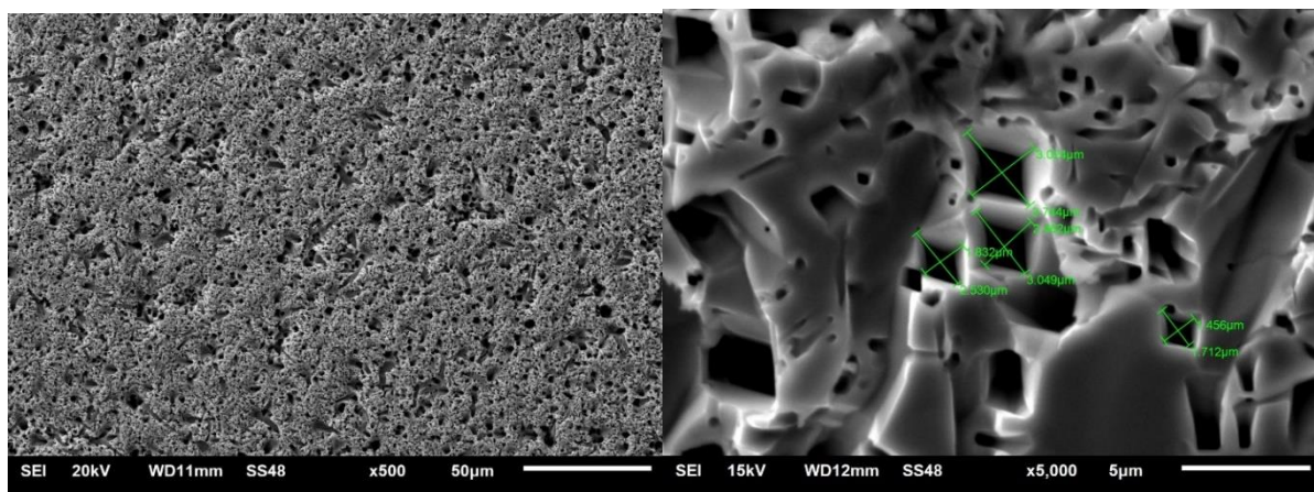
Рис.1. Изображения (РЭМ) пористой структуры на поверхности германия.
