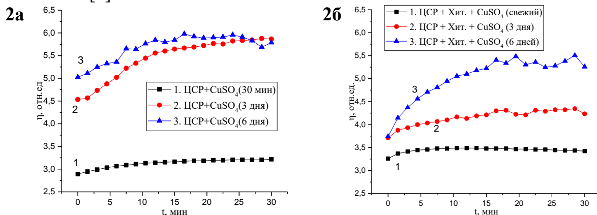
Рис. 2. Зависимость относительной вязкости ЦСР/CuSO 4 (а) и ЦСР/ХЗ/CuSO 4 / (б) гидрогелей от времени: 1 – 30 мин после смешения компонентов, 2 – через 3 дня, 3 – через 6 дней. Объёмы добавляемых ХЗ и CuSO 4 составляют 0,02 мл на 1 мл ЦСР
