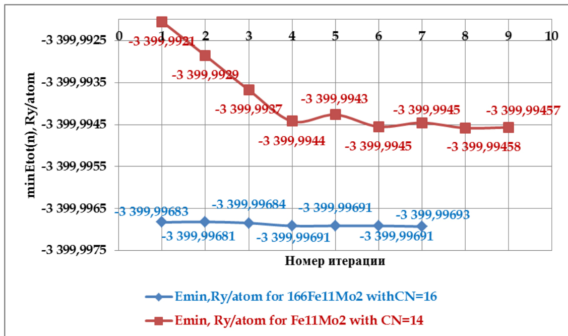
Рис.1. Сравнение зависимостей E_{min}(n) , Ry/atom для разных конфигураций фиксированного состава x((Mo)=0,154 \mu - фазы 166Fe1Fe6Mo2 Fe2Fe2 (Mo CN=16) и 166Fe1Fe6Fe2Fe2Mo2 (Mo CN=14) при n=1 \div 2 dE=10E(-7) Ry/cell, dF=1,0 mRy/au k=2000 ; при n=3 \div 9 dE=10E(-8) , dF=0,5 mRy/au k=5000
