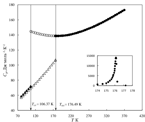
Рис. Температурная зависимость сглаженных значений теплоемкости 4-метилдиоксолана-1,3 при давлении насыщенного пара
