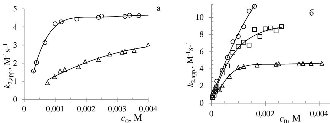
Рис. Зависимость k_{2,app} , \text{M}^{-1}\text{s}^{-1} реакций пероксигидролиза NPDEP от концентрации ПАВ (вода, pH 11.0, 25°): а – ПАВ: I (o), II ( \Delta ); б – ПАВ: III (o), V ( \square ), I ( \Delta ).
