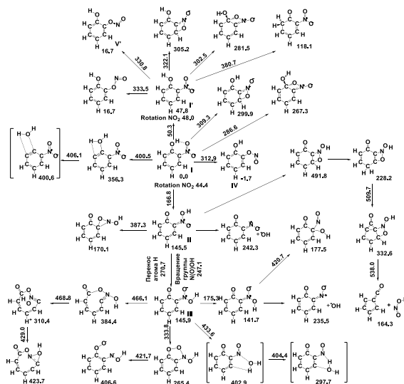
Рис. 1 – Схема термического распада 2-нитрофенола, полученная методом V3LYP/6-31+G(2df,p)*. Рис. 2 – Схема термодеструкции 2-нитрофенола, полученная методом QM_N3*.
