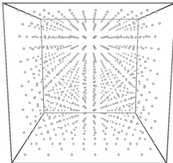
Рис. 1. Начальная конфигурация моделируемой системы.
