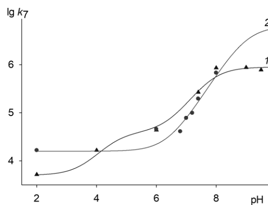
Рис. 2. Зависимости \lg k_7 от рН для аскорбиновой кислоты (1) и эпикатехина (2). Точки – эксперимент, линии – расчет.
