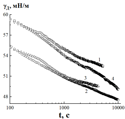
Рис. 2. Изменение динамического поверхностного натяжения растворов солей ГК от времени. 1 – ГН; 2 – ГНГК+пэг-6000; 3 – ГНГК+гуанидин; 4 – ГНГК+пэг-6000+гуанидин. СПАВ = 0,8%.
