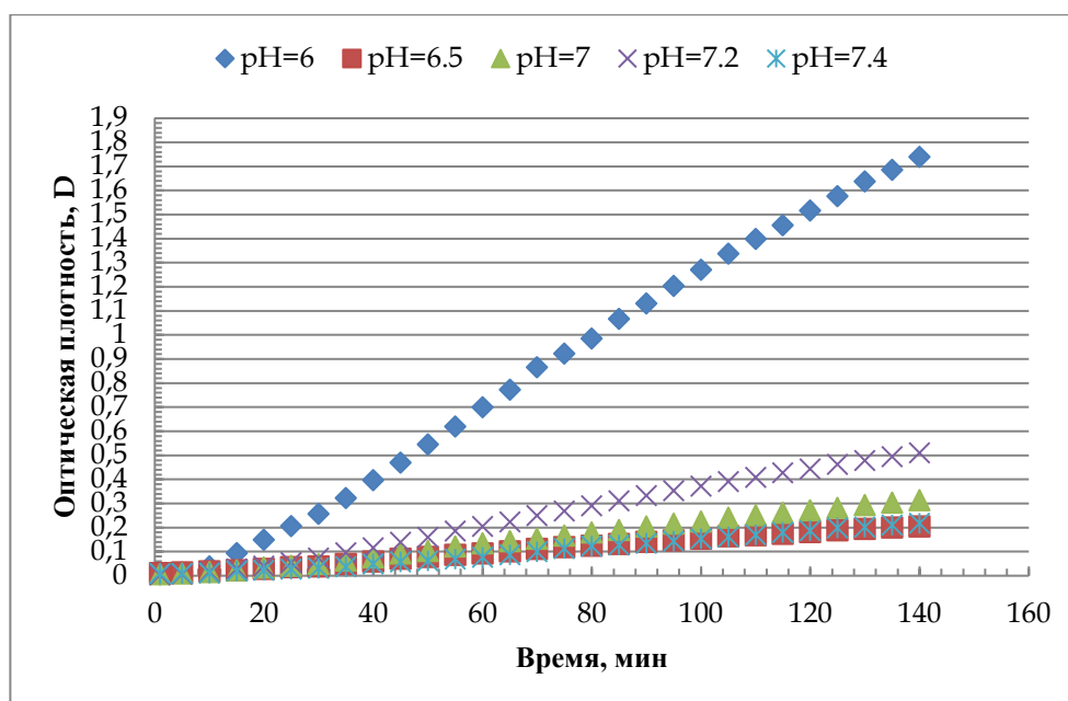
Рис. 1. Влияние pH на оптическую плотность
