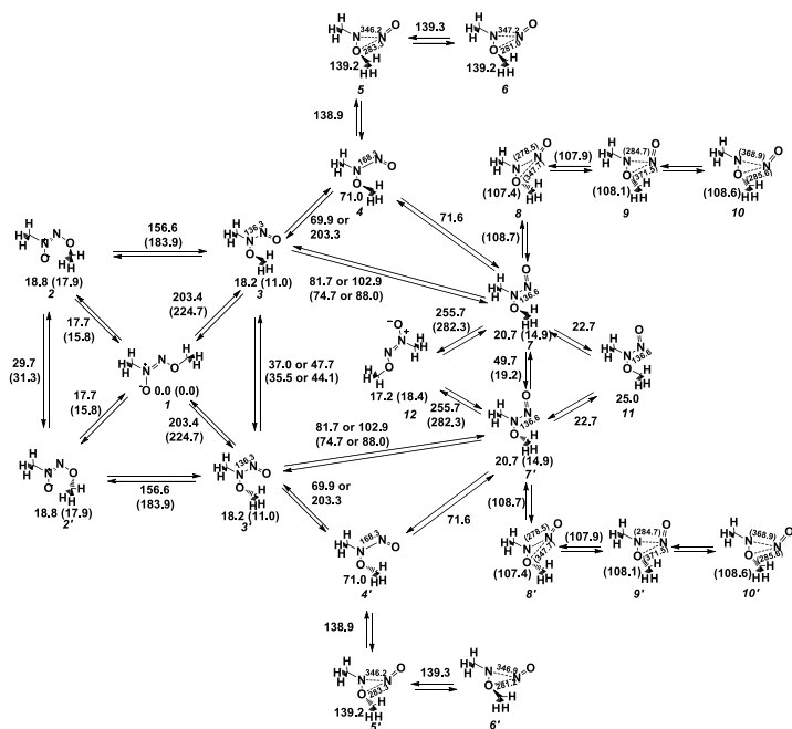
Рис. 1. Схема отщепления оксида азота от N-метил-N'-метоксидазена-N-оксида ( 1 ) (по данным PBE/L11 и (в скобках) V3LYP/6-31G(2df,p)). Здесь и на рис. 2 относительные энтальпии образования переходных состояний (над-под стрелками), реагентов и продуктов (под соединениями) реакций в кДж/моль. За ноль принята энтальпия образования соединения 1 . «Ог» – означает альтернативные пути, отличающиеся направлением поворота групп.
