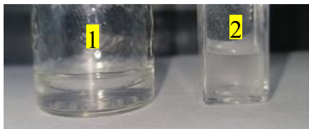
Рис. 1 Фото образцов ЦСР (1 мл) с различным содержанием KBr: 0.0300 мл (1), 0.0325 мл (2) через 20 мин после приготовления (слева направо)
