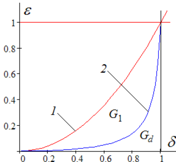
Рисунок. Кривая 1 – \varepsilon = \delta^2 , кривая 2 – \varepsilon = 0.1\delta^2/(1.1 - \delta^2) .
