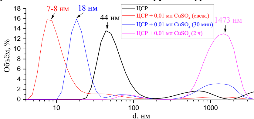
Рис. 3. Распределение агрегатов по размерам в ЦСР после добавления сульфата меди в зависимости от времени
