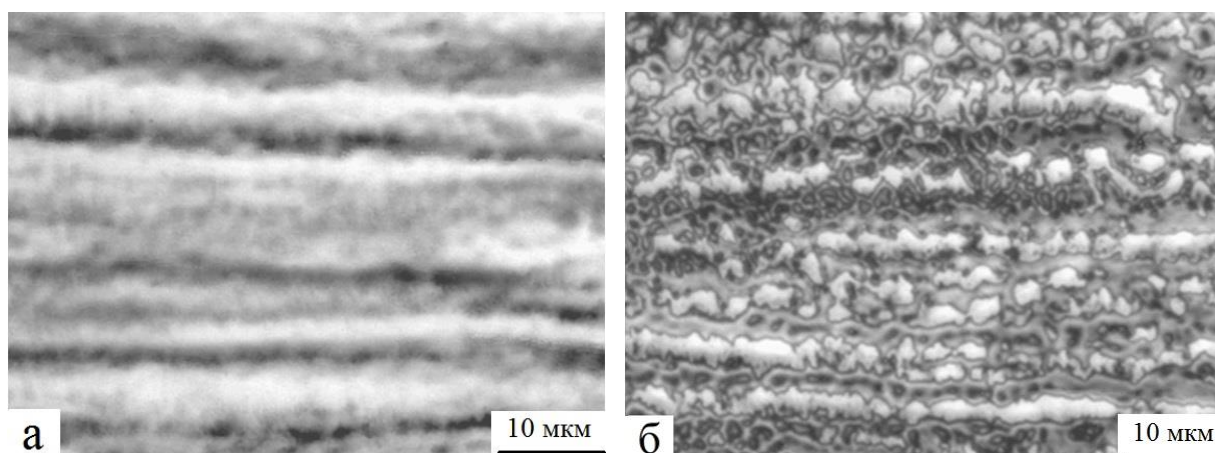
Рис. 1. Микрофотографии поверхности нержавеющей стали 12X18H10T: а) исходная поверхность; б) после обработки сканирующим пучком Nd:YAG-лазера в вакуумной камере (плотность энергии в импульсе – 1,1 Дж/см 2 , скорость сканирования – 1,0 мм/с)
