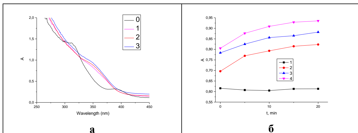
Рис. 2. Электронные спектры образцов с различным содержанием KBr: 0 – ЦСР, 1 - 0.0275, 2 - 0.030, 3 - 0.0325 мл /1 мл ЦСР – а; кинетическая зависимость оптической плотности (A) на длине волны 350 нм для образцов с различным содержанием KBr: 2 - 0.0250, 2 - 0.0275, 3 - 0.030, 4 - 0.0325 мл /1 мл ЦСР – б
